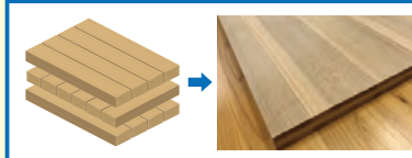
「強く美しい建築材料」スギ桎目板CLT(直交集成板)パネル
