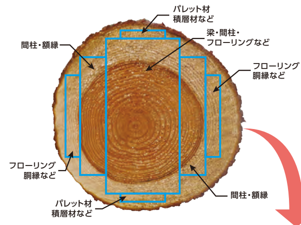
大径材を活かす新たな木取りの提案(丸太末口直径44cm)
